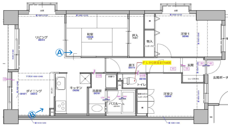
リフォーム後の平面図
